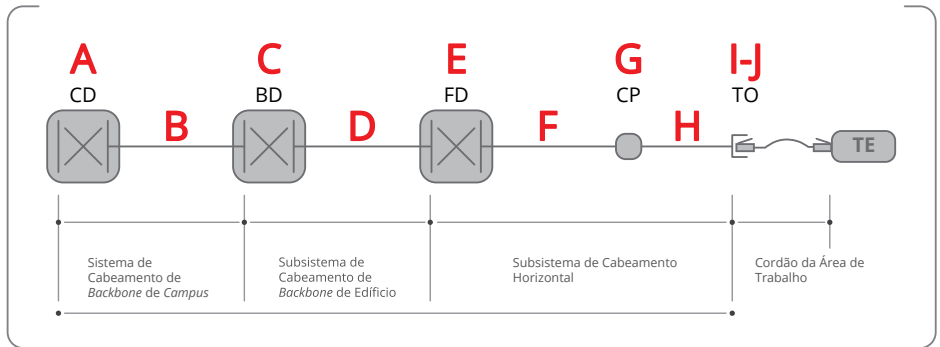
Estrutura do cabeamento em edifícios corporativos de acordo com a norma ABNT14565.
